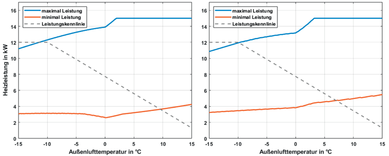
Abb. 5: Leistungsbereich der EU13L je nach Außenlufttemperatur bei 5K Spreizung und 85 % Luftfeuchte (links: 35 °C Vorlauftemperatur / rechts: 55 °C Vorlauftemperatur) mit empfohlener Leistungskennlinie nach EN 14825.
