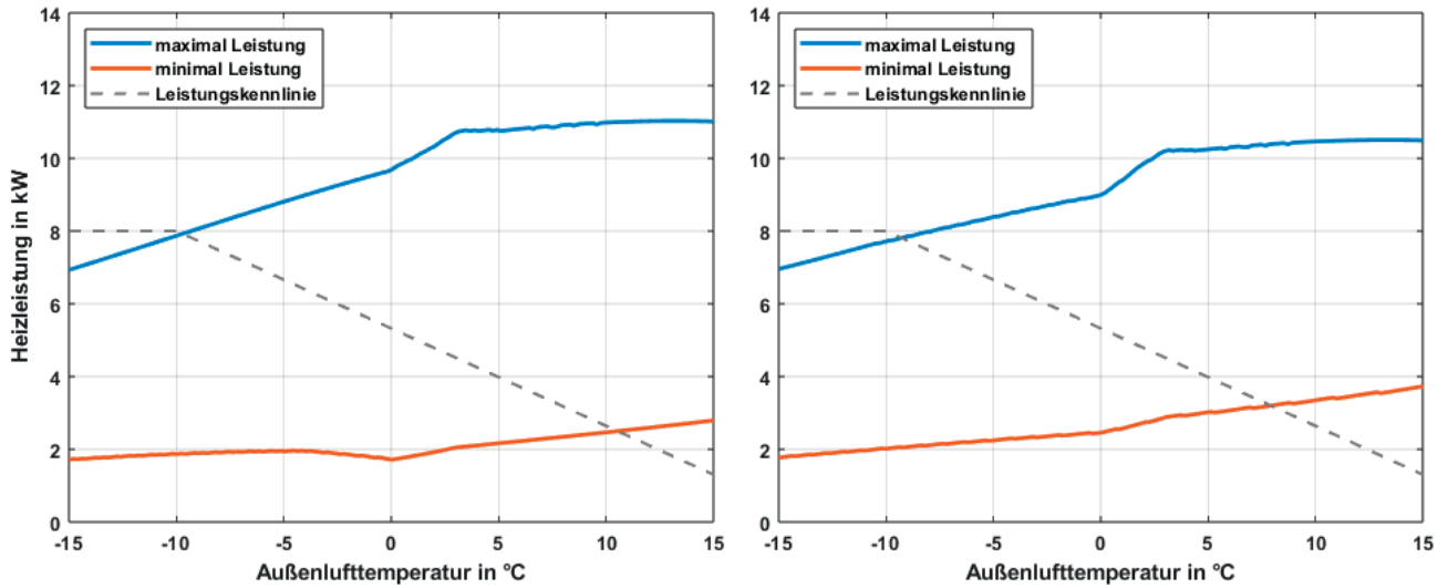
Abb. 1: Leistungsbereich der EU08L je nach Außenlufttemperatur bei 5K Spreizung und 85 % Luftfeuchte (links: 35 °C Vorlauftemperatur / rechts: 55 °C Vorlauftemperatur) mit empfohlener Leistungskennlinie nach EN 14825.
