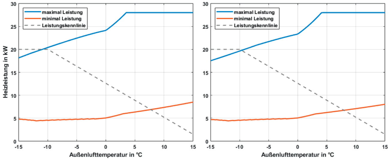
Abb. 9: Leistungsbereich der EU13L je nach Außenlufttemperatur bei 5K Spreizung und 85 % Luftfeuchte (links: 35 °C Vorlauftemperatur / rechts: 55 °C Vorlauftemperatur) mit empfohlener Leistungskennlinie nach EN 14825.
