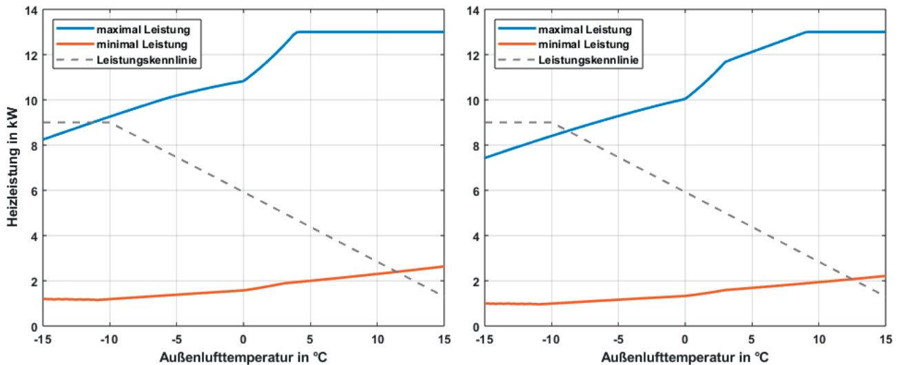
Abb. 3: Leistungsbereich der EU10L je nach Außenlufttemperatur bei 5K Spreizung und 85 % Luftfeuchte (links: 35 °C Vorlauftemperatur / rechts: 55 °C Vorlauftemperatur) mit empfohlener Leistungskennlinie nach EN 14825.
