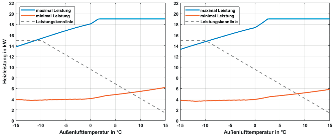
Abb. 7: Leistungsbereich der EU15L je nach Außenlufttemperatur bei 5K Spreizung und 85 % Luftfeuchte (links: 35 °C Vorlauftemperatur / rechts: 55 °C Vorlauftemperatur) mit empfohlener Leistungskennlinie nach EN 14825.
