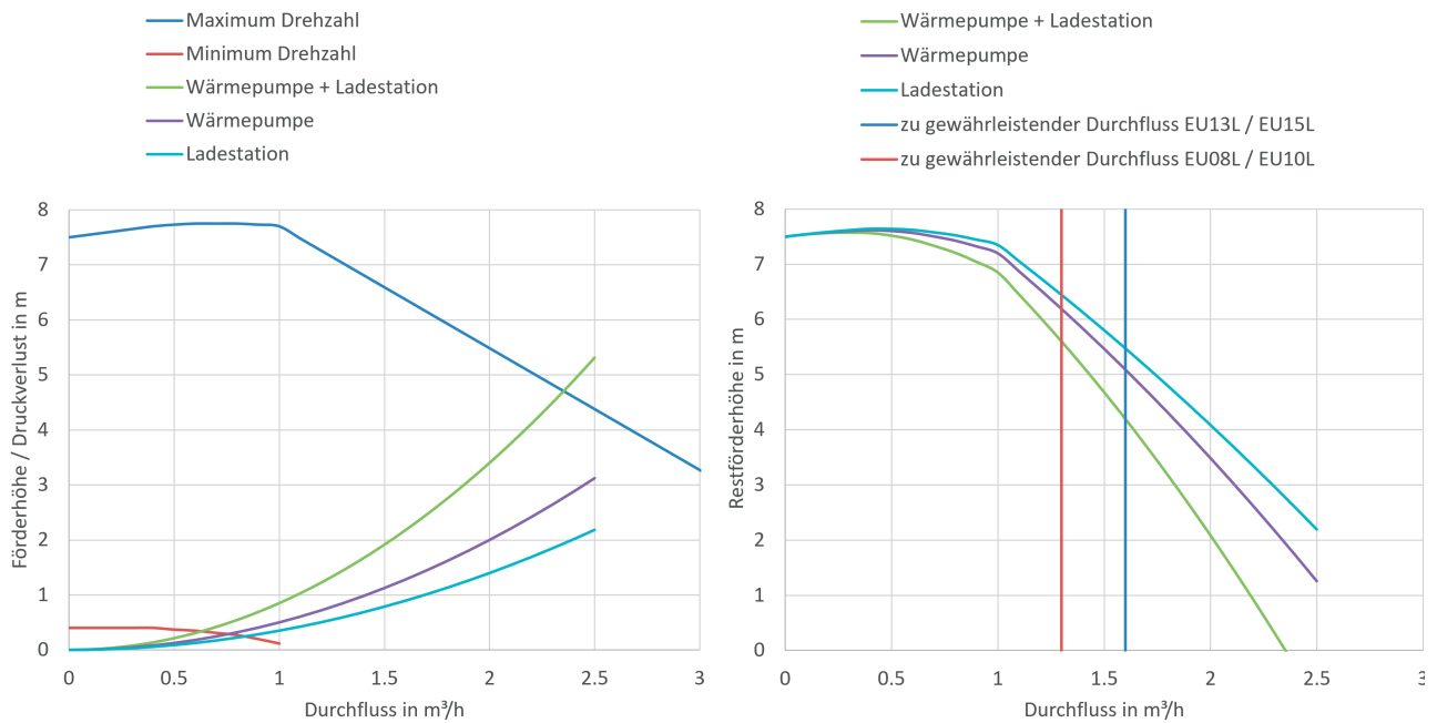
Abb. 11: Pumpenkennlinie, Anlagenkennlinie und Restförderhöhe EU08L, EU10L, EU13L, EU15L
