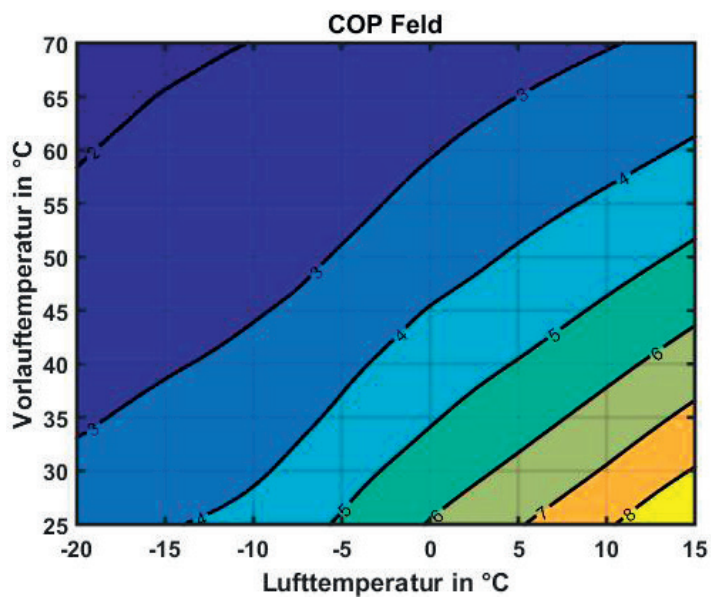
Abb. 6: EU13L bei 9kW Heizleistung
