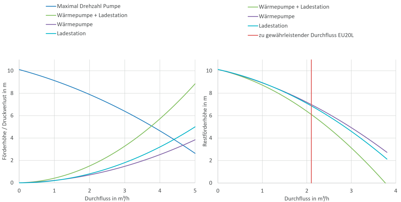
Abb. 12: Pumpenkennlinie, Anlagenkennlinie und Restförderhöhe EU20L
