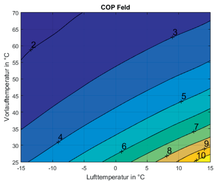
Abb. 4: EU10L bei 6kW Heizleistung
