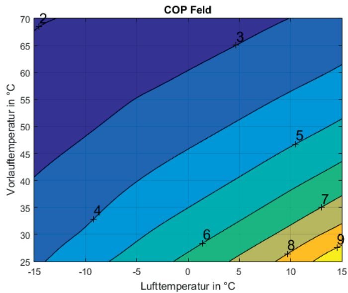
Abb. 10: EU20L bei 14kW Heizleistung
