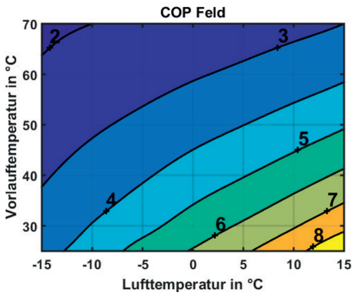
Abb. 8: EU15L bei 11kW Heizleistung
