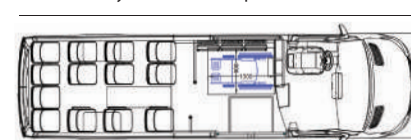
Novus Cityline LW - 16 Sitzplätze + Rollstühle
