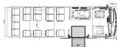
Novus City V7 - 18 Sitzplätze + 1 Rollstuhlplatz
