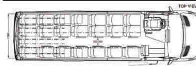
Ecoline L - 22 Sitzplätze+ 3 Rollstühle
