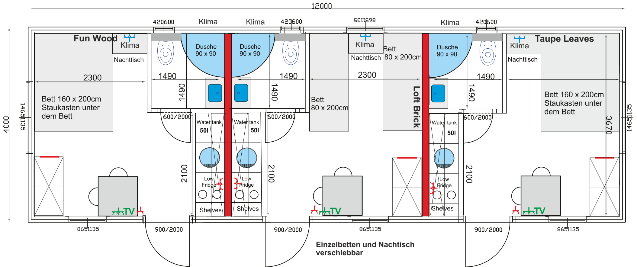
Apartmenthaus mit 3 Einheiten von 12 x 4m bis 14 x 4m
