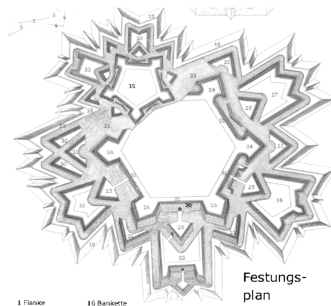
Grundriss einer Bastionsfestung Quelle: Wikimedia Commons (Public Domain).
