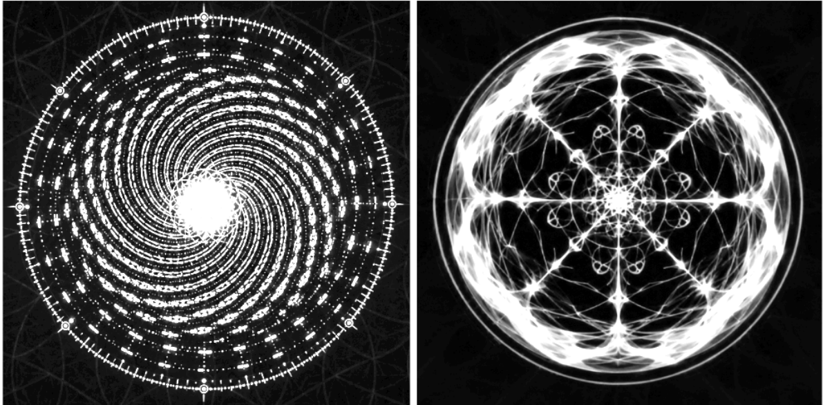
Kymatische Klangfiguren zweier Frequenzen Künstlerische Illustration, erstellt mit Unterstützung künstlicher Intelligenz
