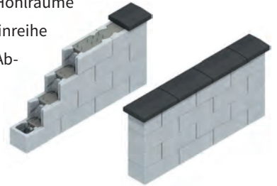
Der Aufbau einer Schalungssteinmauer
