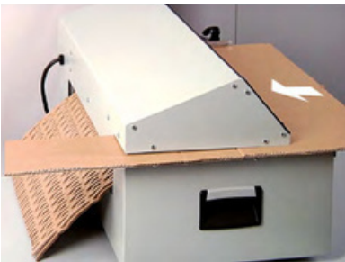
Kullanımı kolay, ayarlanabilir çalışma genişliği. Giriş boğazından daha büyük boyutlu kartonları otomatik olarak keser.
