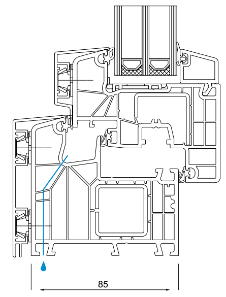
ENTWÄSSERUNG NACH UNTEN
