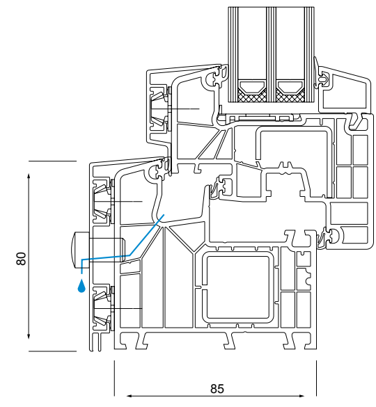
ENTWÄSSERUNG DURCH ALUSCHALE
