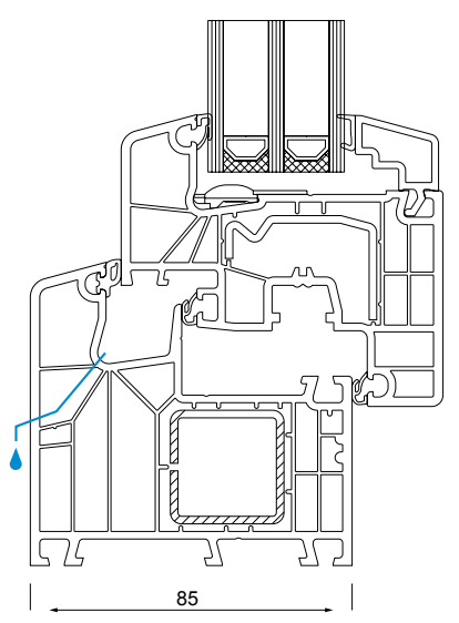
ENTWÄSSERUNG NACH VORNE
