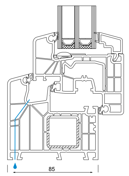
ENTWÄSSERUNG NACH UNTEN
