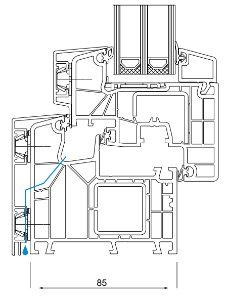
ENTWÄSSERUNG NACH VORNE
