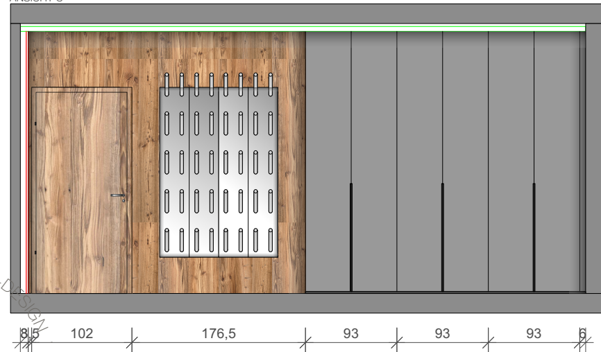
ANSICHT C
