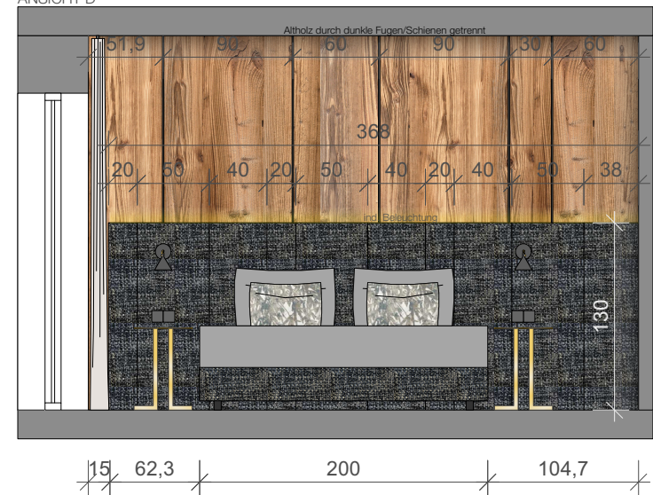
ANSICHT D
