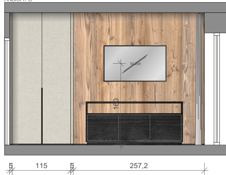
ANSICHT B
