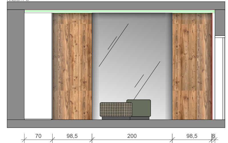
ANSICHT B
