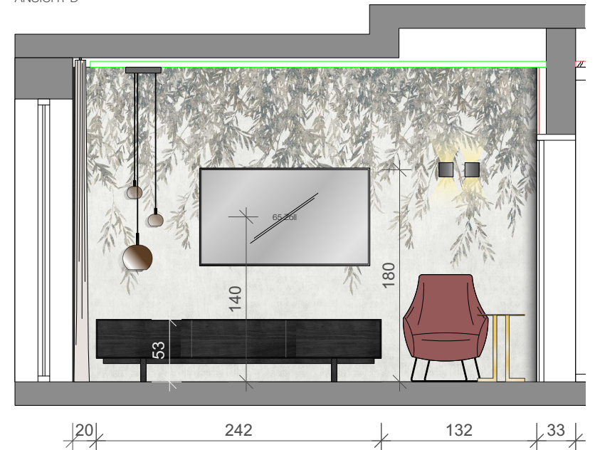
ANSICHT D
