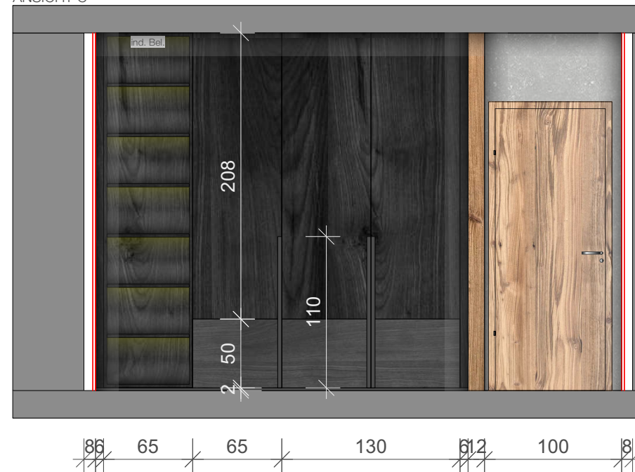
ANSICHT C
