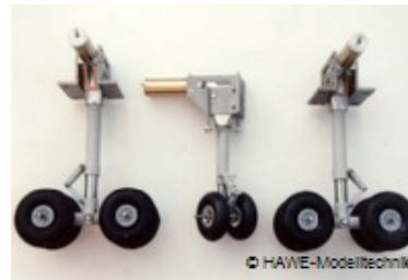
Airbus A300 Spannweite: 3,00 m Gewicht: 19 kg
