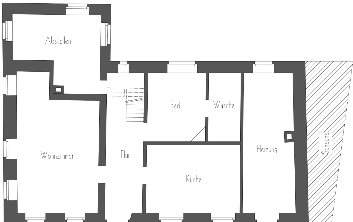
Römerstraße 9 - ERDGESCHOSS
