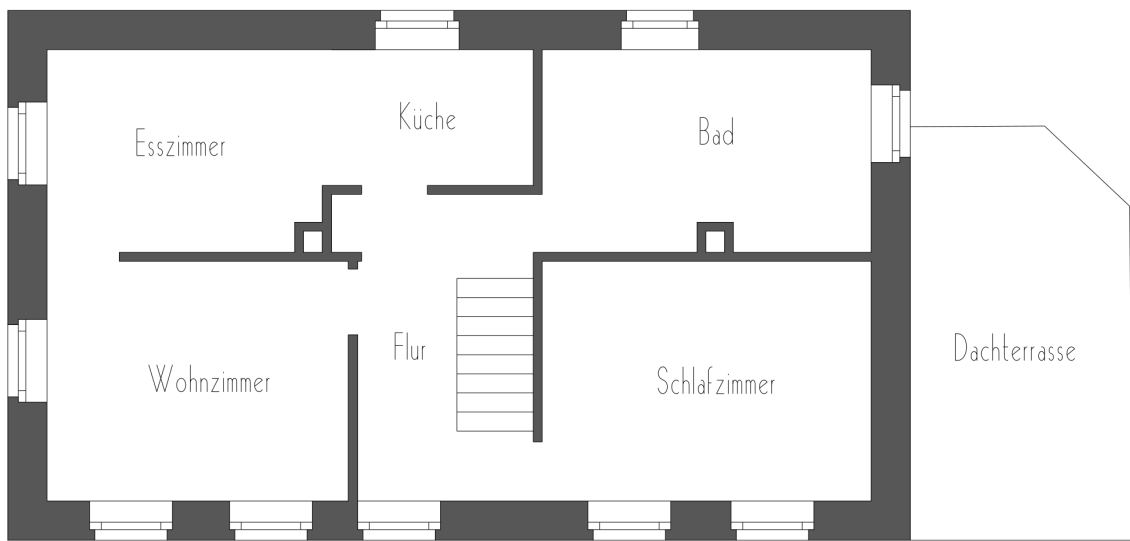
Römerstraße 8 - OBERGESCHOSS
