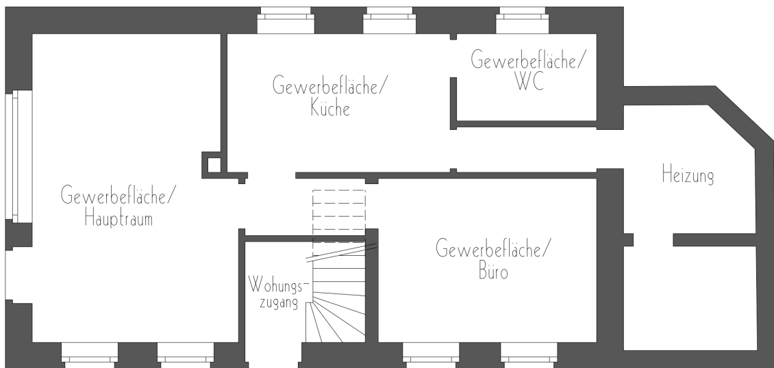
Römerstraße 8 - ERDGESCHOSS
