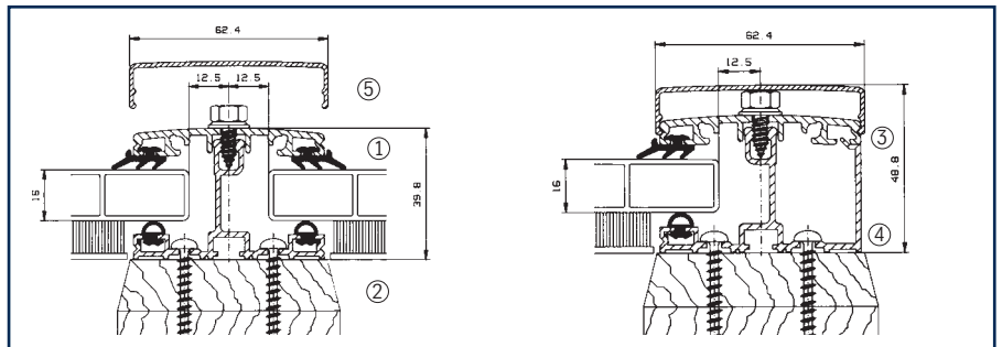
ALWO®-Komplettsystem 16, Ausführung pressblank inkl. Dichtungsprofilen bestehend aus:
