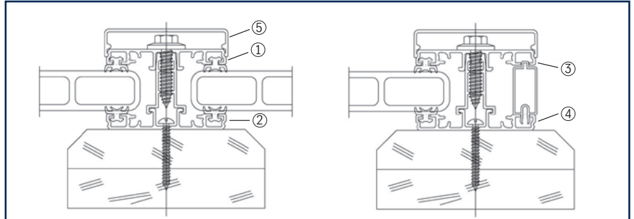
ALWO®-THERMOSPROSSE 5562, Ausführung pressblank inkl. Dichtungsprofilen bestehend aus:
