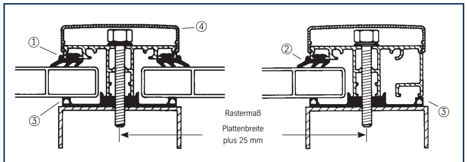
ALWO®-Oberprofilssystem 16/20/32, Ausführung pressblank inkl. Dichtungsprofilen bestehend aus:
