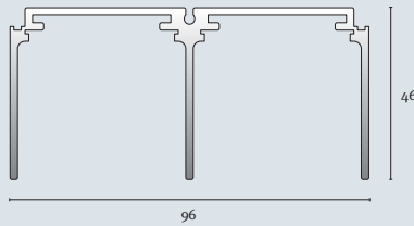
Deckenschiene zweiläufig
