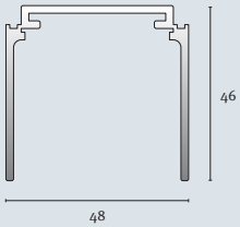
Deckenschiene einläufig
