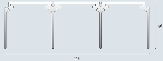
Deckenschiene dreiläufig
