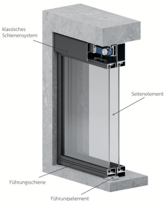
Ansicht bei Deckenmontage mit Seitenteil
