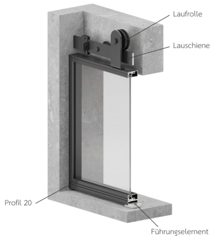
Ansicht bei Wandmontage
