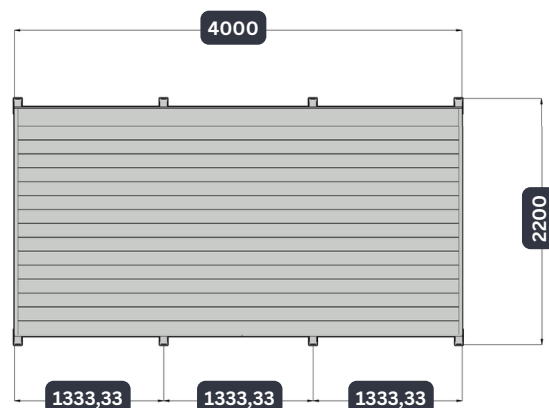
Bodenansicht
