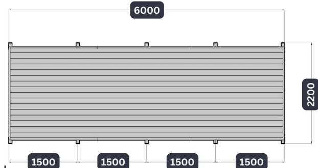
Bodenansicht
