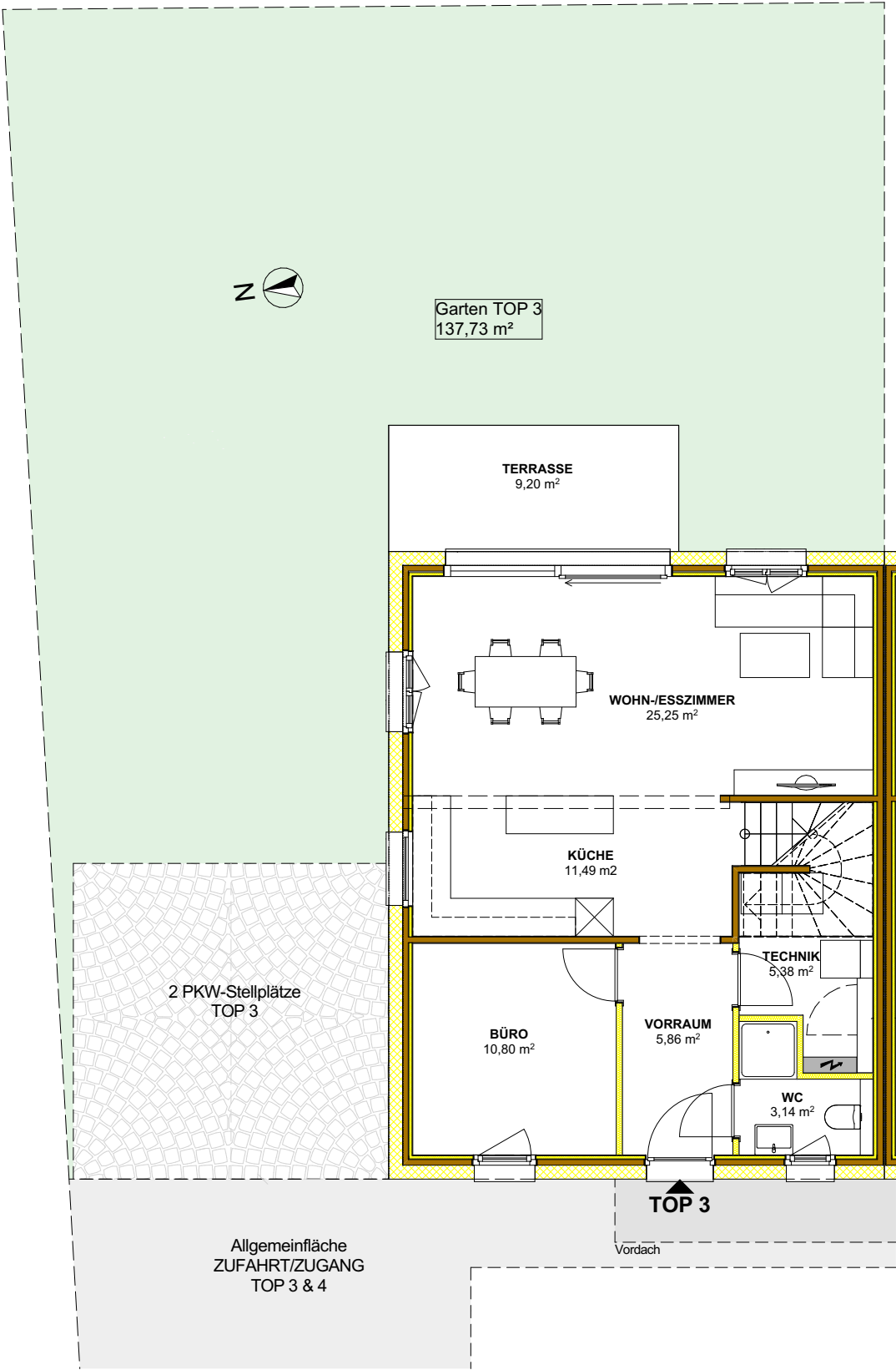
ERDGESCHOSS
