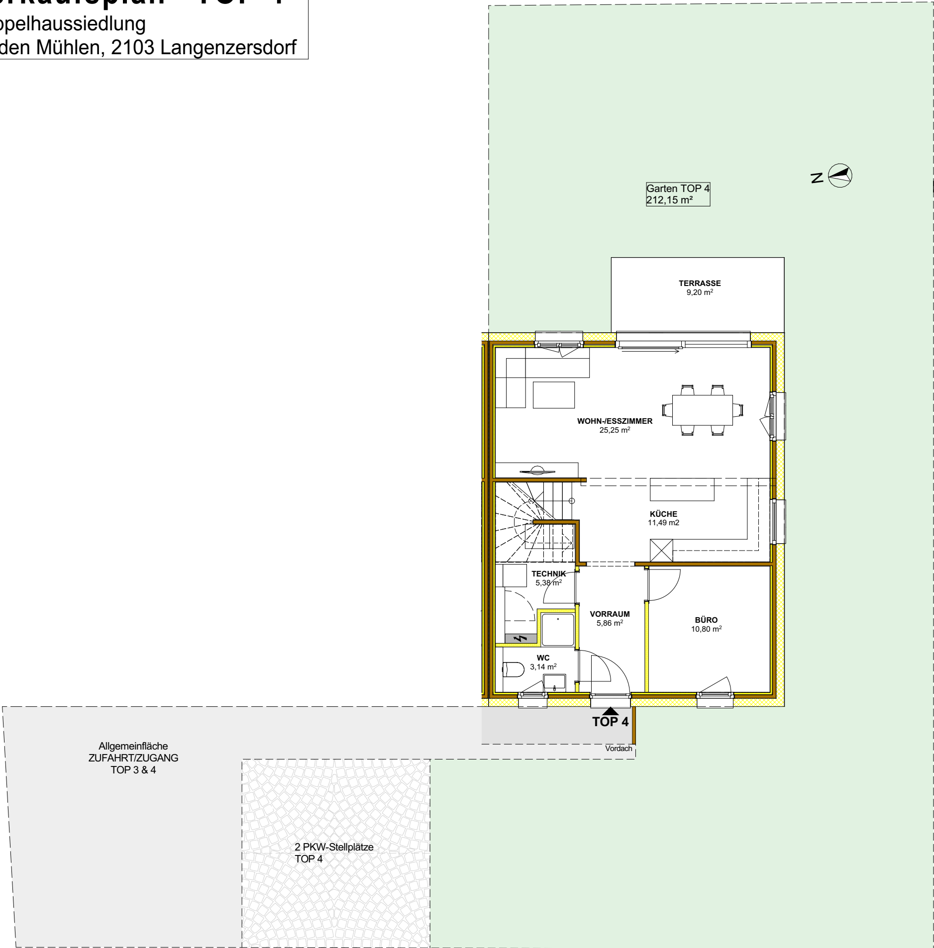
ERDGESCHOSS
