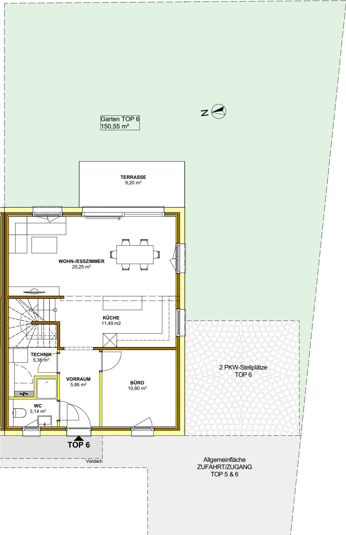
ERDGESCHOSS
