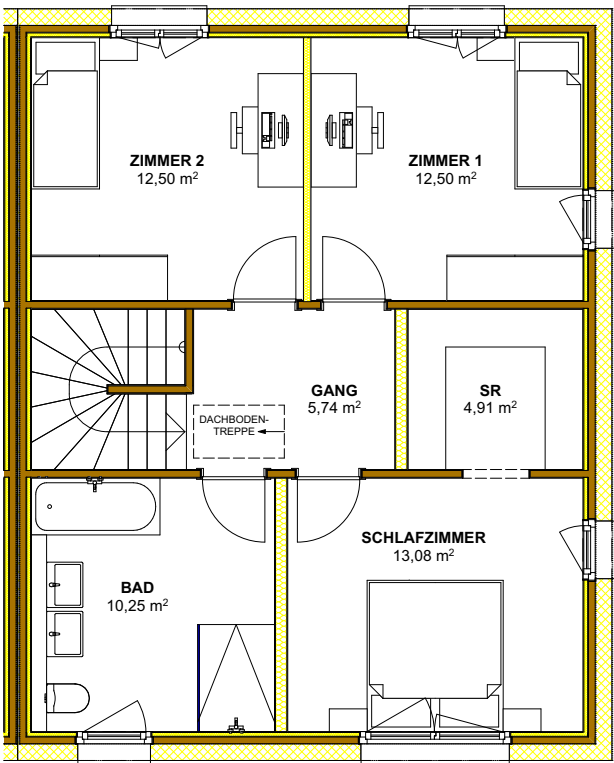
OBERGESCHOSS
