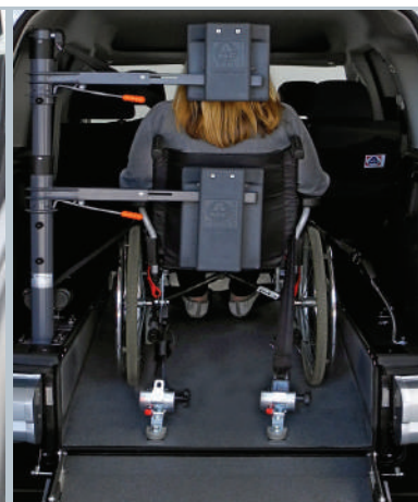
Le véhicule est équipé de l'appui-tête et du support dorsal FUTURESAFE
