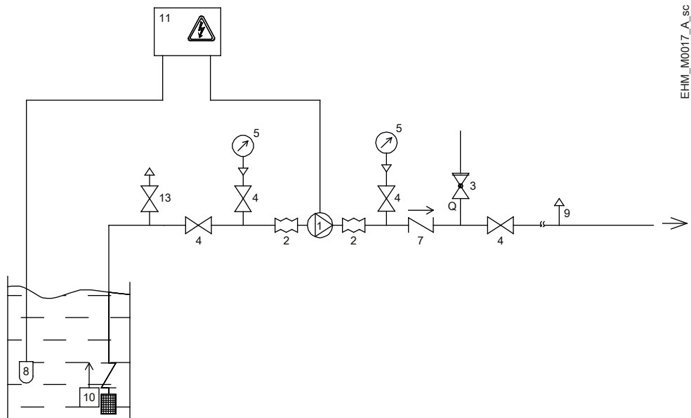
Abb. 2: Installation im Saugbetrieb
