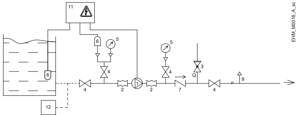
Abb. 1: Anordnung mit positivem Zulaufdruck
