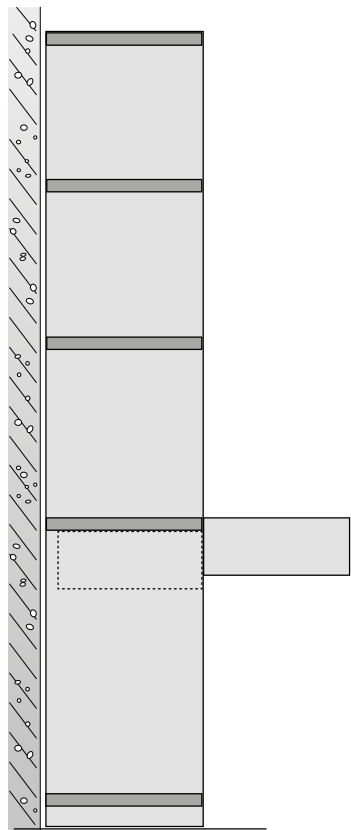
Balda elevable para estantería con paneles W3 — (B3WTAL...48) Unión a ras con el estante de 2,8 cm
