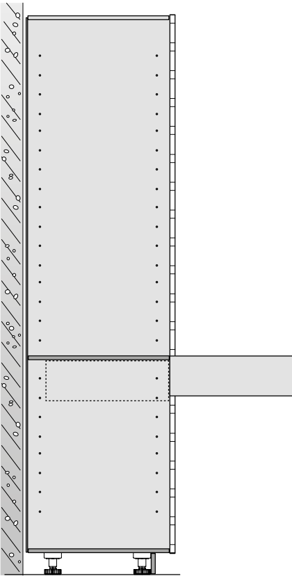
Balda elevable para columna (HTAL...)
