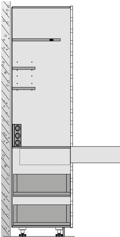
Balda elevable en lugar de balda extraíble (ANTALVF)
