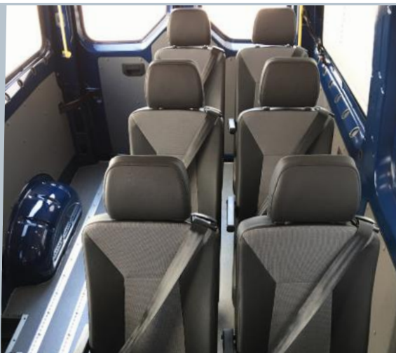
Les sièges Smartseats peuvent être disposés de manière flexible dans l'habitacle selon les besoins
