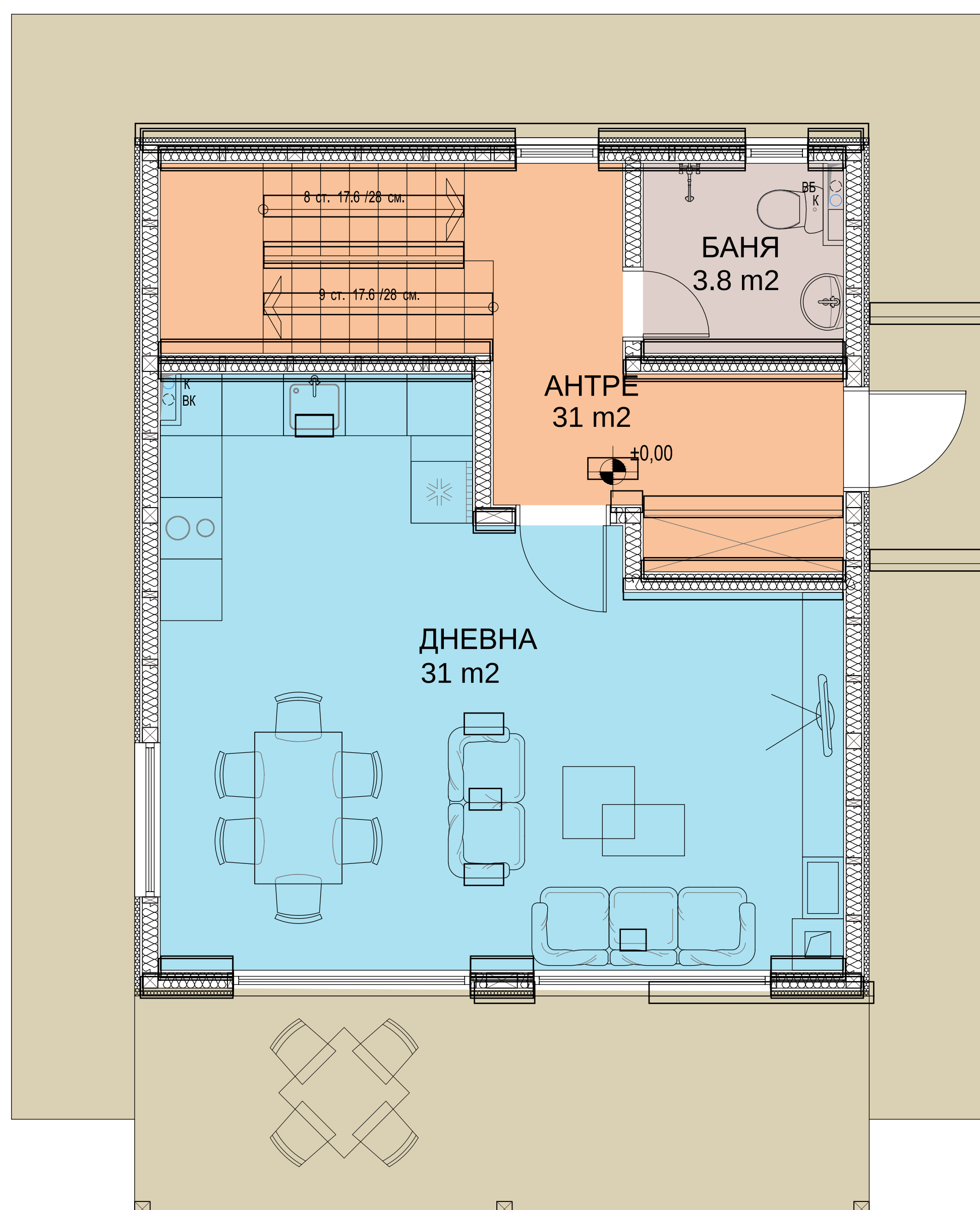
РАЗПРЕДЕЛЕНИЕ 1-ви ЕТАЖ КОТА ±0.00 ЗП = 75,07 м²
