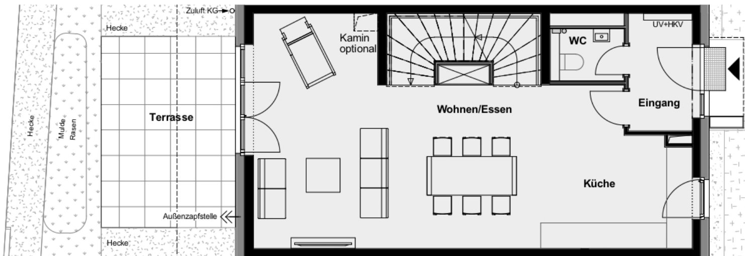
Erdgeschoss
