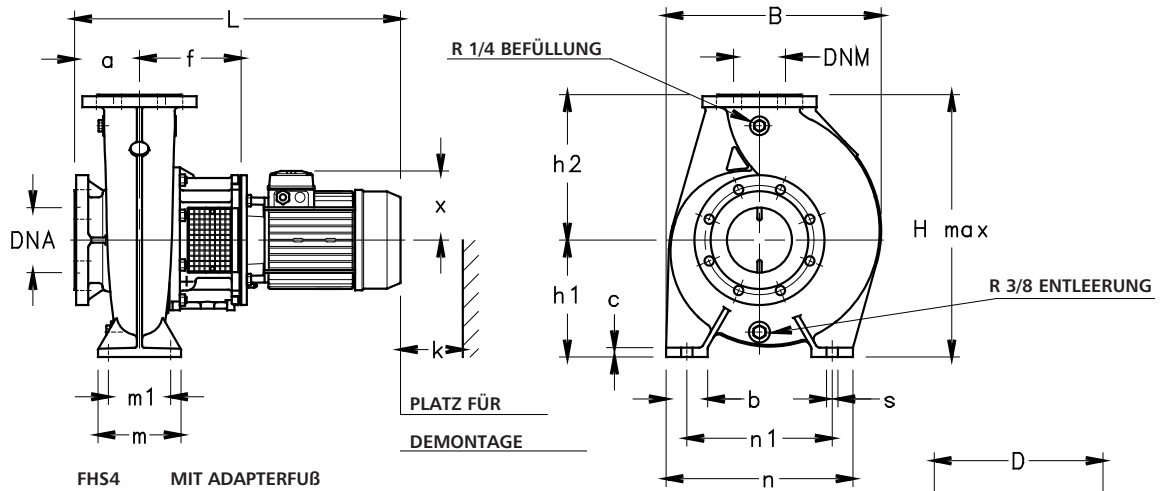
FLANSCHABMESSUNGEN
