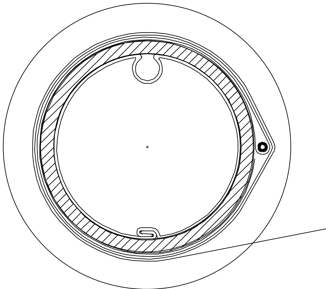
Bandverlauf Wickelrolle
