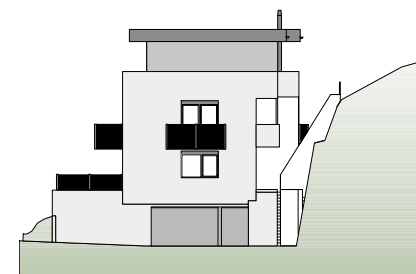
Ansicht Nord-Ost
